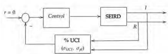
Figura 2. Sistema realimentado (lazo cerrado) que permite la disminución de ocupación de camas de UCI.
